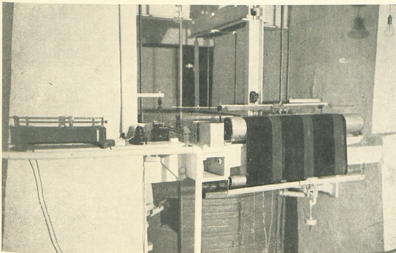
Partie inférieure du séismographe de Quervain-Piccard : mécanisme d'inscription.
