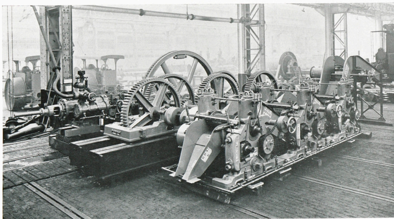
ENSEMBLE DE 3 MOULINS A CANNES DE 406 × 610 AVEC MOTEURS A VAPEUR POUR DISTILLERIE
