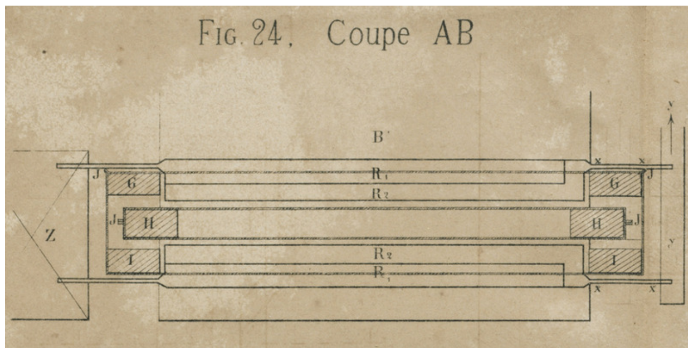
Figure 24 : Cheminée de dessiccation et de réfrigération simultanées (toile)
