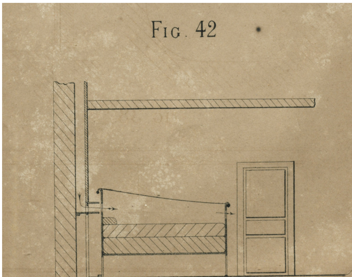
Figure 42 : Lit ventilé par un courant d'air atmosphérique chaud et humide
