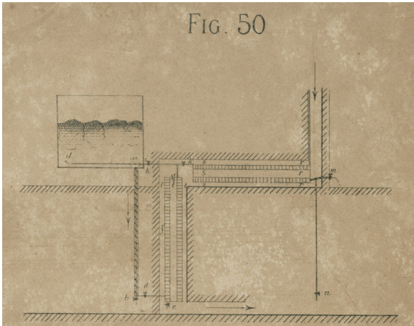
Figure 50 : Schéma d'une installation à circulation d'eau froide. Réservoir à glace et poëles réfrigérants
