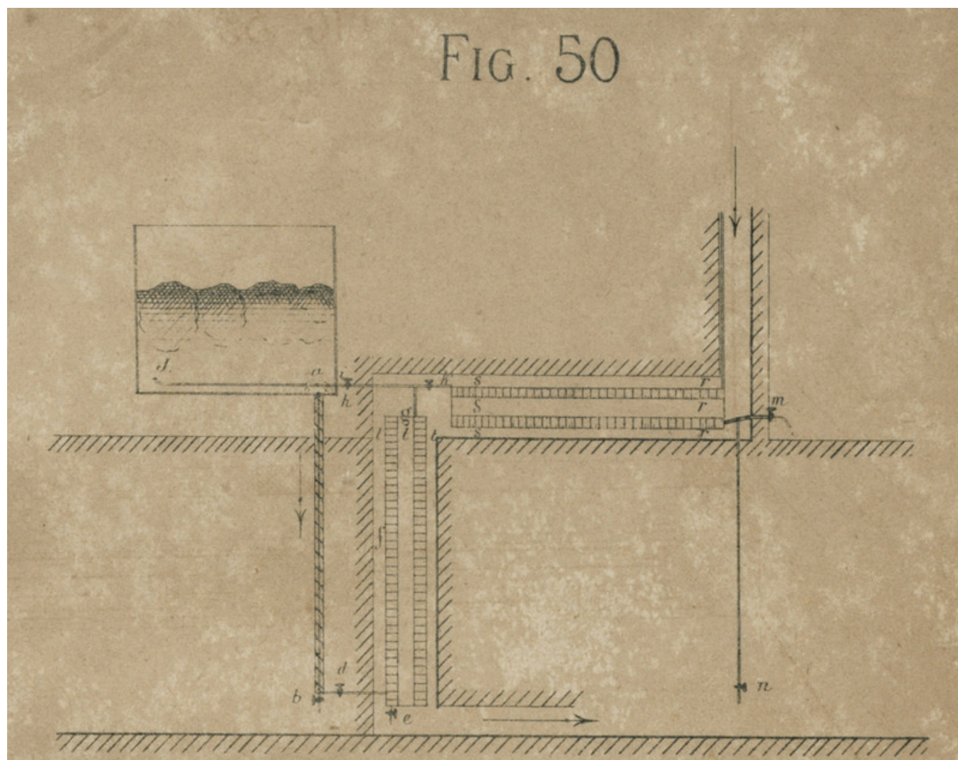
Figure 50 : Schéma d'une installation à circulation d'eau froide. Réservoir à glace et poêles réfrigérants
