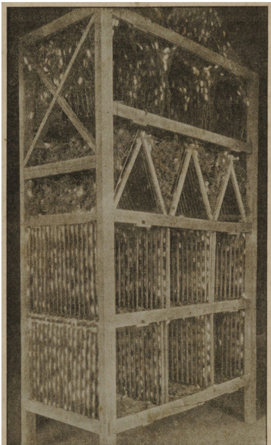
Vue d'ensemble d'un bâti comprenant des claies coconnières Davril, un étage de claies coconnières prismatiques de Nanisana et trois arceaux en bruyères représentant l'encabanage le plus communément employé.
