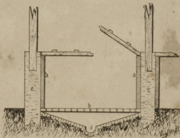
Fig. 2. — Élévation transversale.
