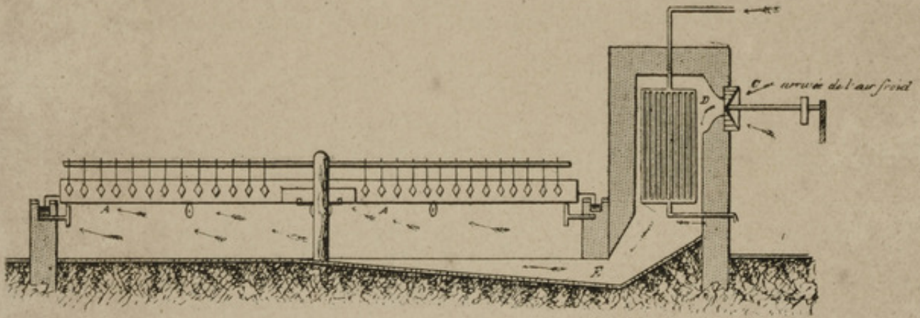
Fig. 1. — Coupe transversale.
