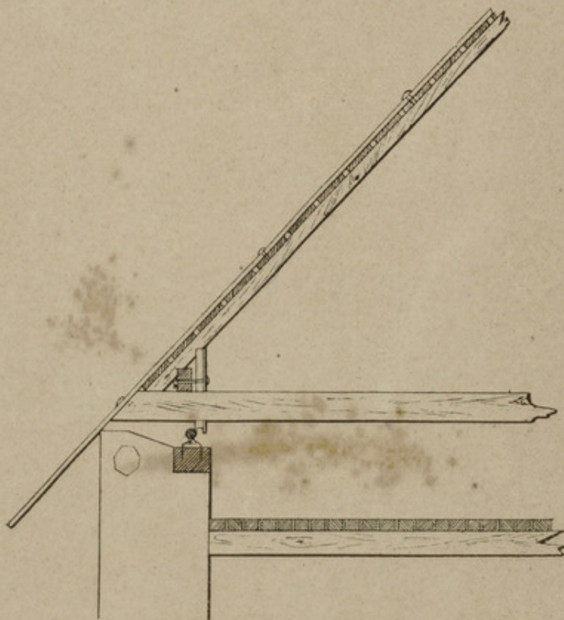
Fig. 2. — Détail de suspension du toit.
