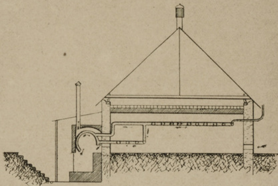
Fig. 1. — Coupe transversale.
