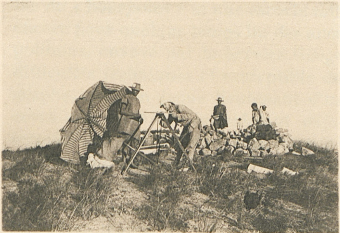
Construction d'un signal géodésique.
