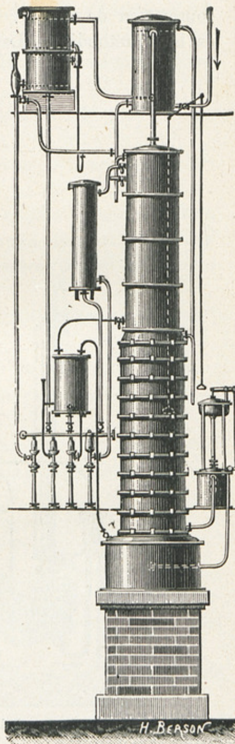
FIG. 78. — Colonne à haut degré (système Barbet).
