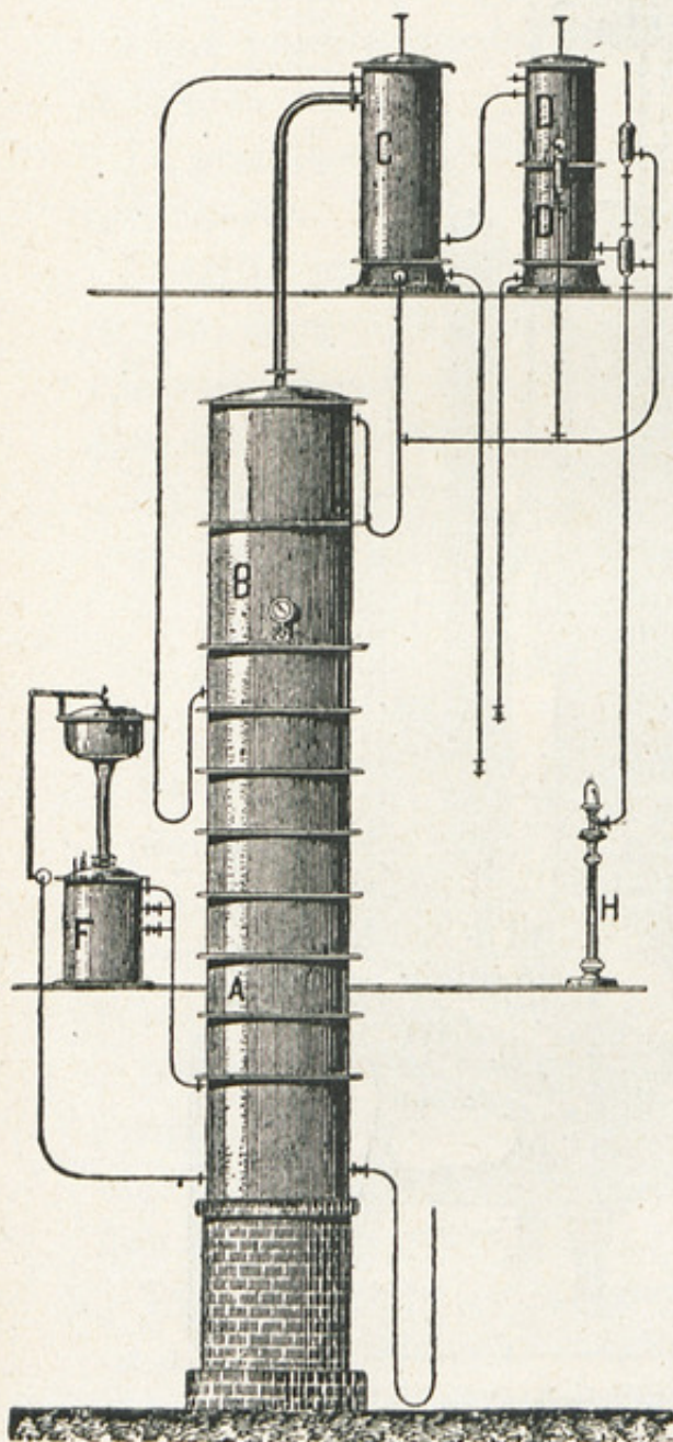
FIG. 77. — Colonne à distiller à haut degré (système Barbet).
