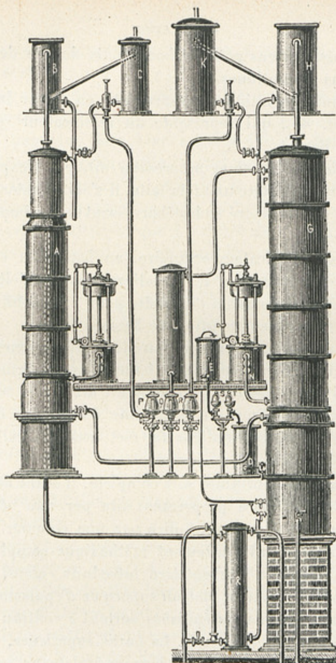
FIG. 82. — Rectification continue (système Barbet).
