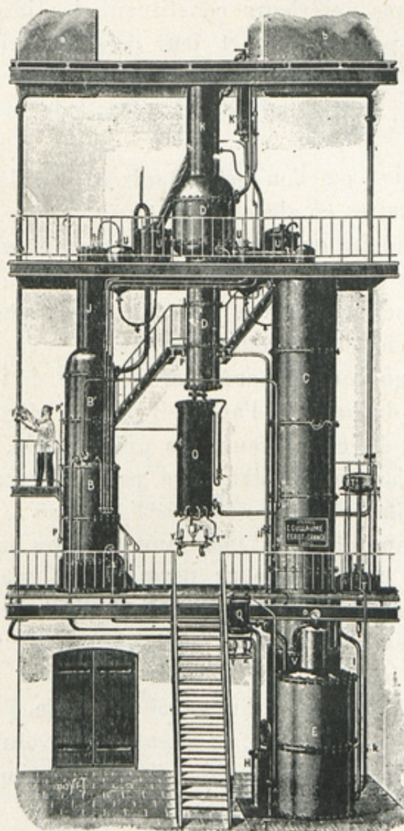
FIG. 83. — Appareil de rectification continue (système Guillaume).
