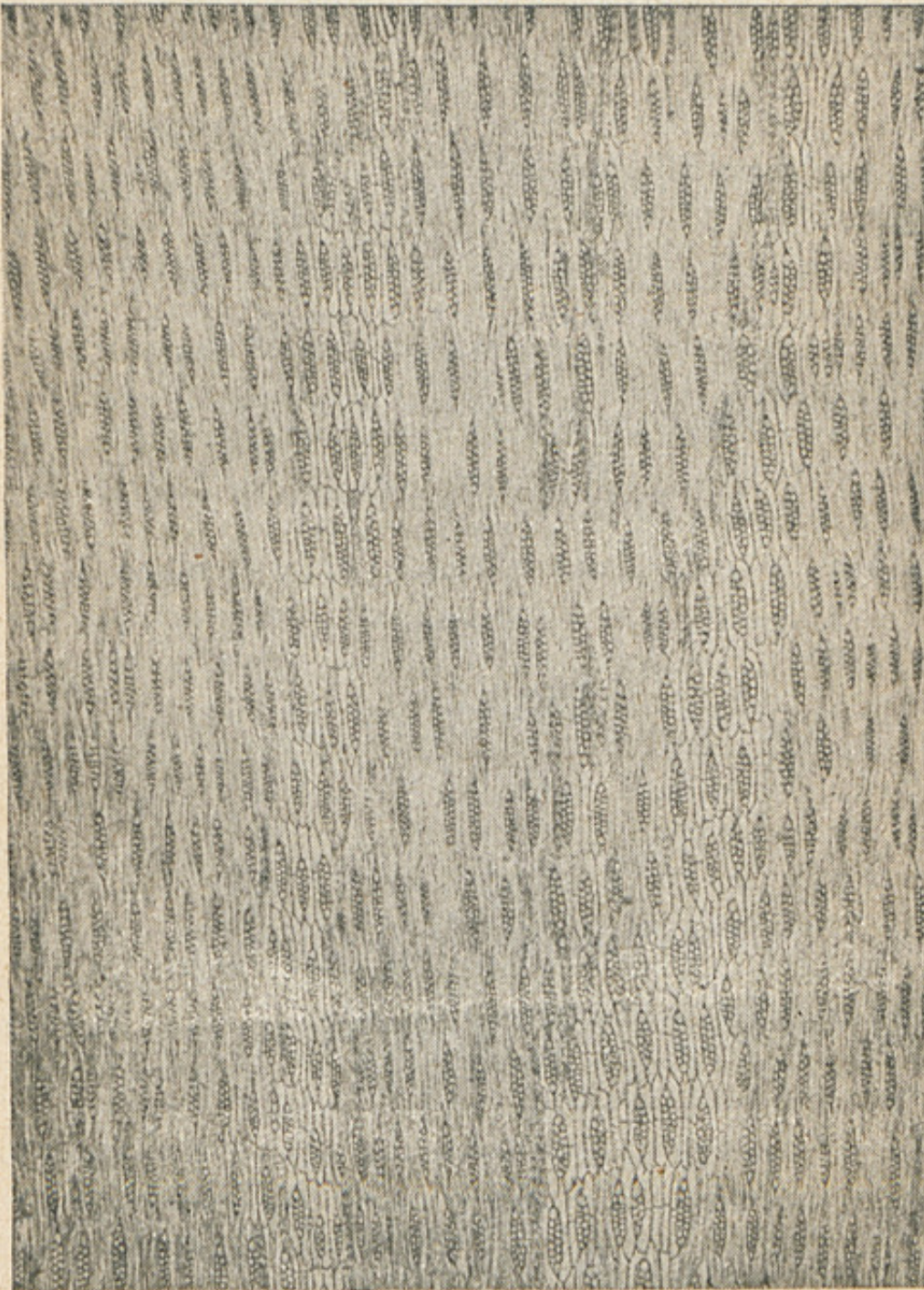
Fig. 19. — SECTION LONGITUDINALE TANGENTIELLE DE BOIS DE Dalbergia Oliveri Gamble (Légumineuses), avec rayons nettement étagés. (Grossissement : 30 diam.)
