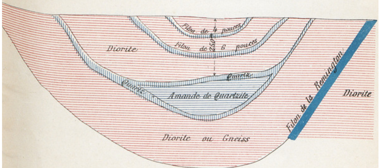
SCHÉMA MONTRANT LE SYSTÈME DU CALLAO
