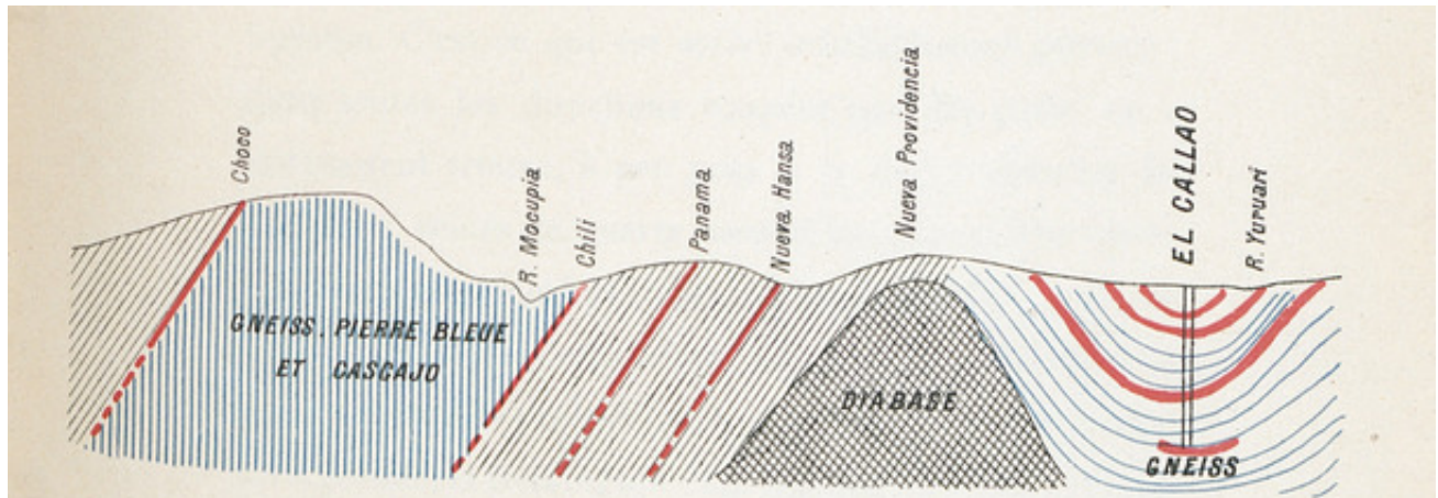
COUPE DU BASSIN, d'après l'Ingénieur N. PAQUET
