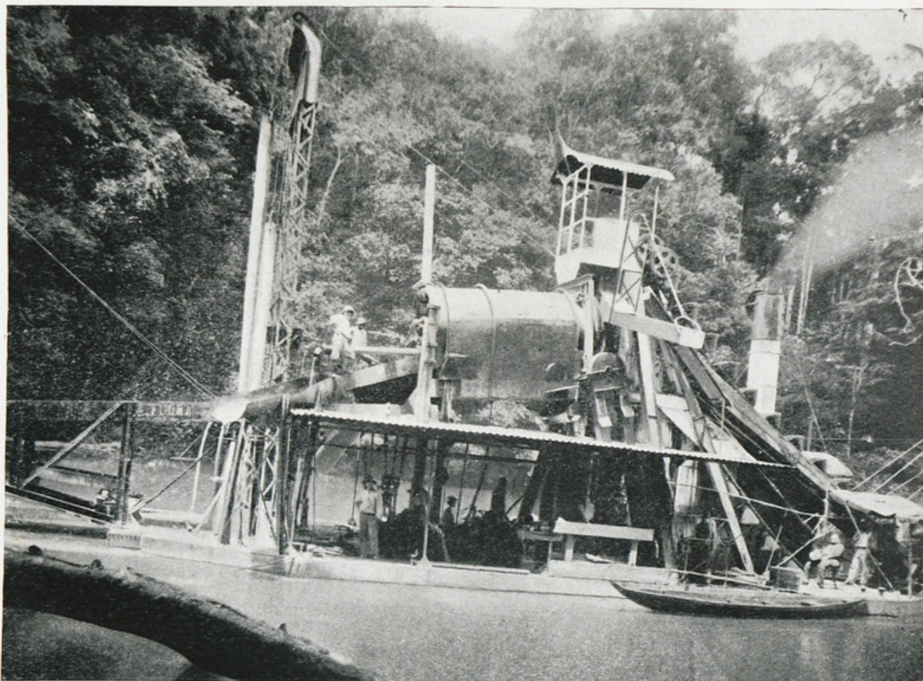
UN CHANTIER D'EXPLOITATION ALLUVIONNAIRE PAR DRAGUE A OR EN FONCTIONNEMENT
